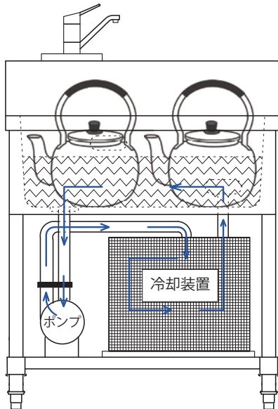
図面 Type-1A バックガード付
