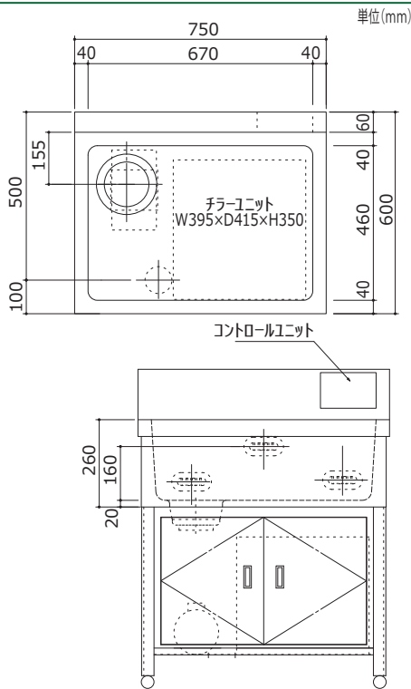
図面 Type-1A バックガード付
