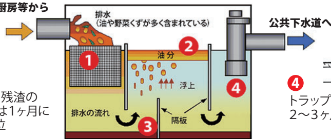
グリストラップを横からみた図
